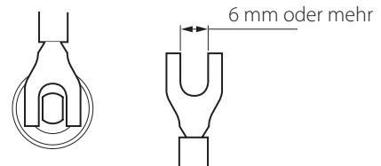
Schnittbild der Schraubklemme
