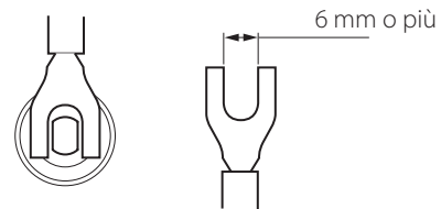
Sezione trasversale del terminale
